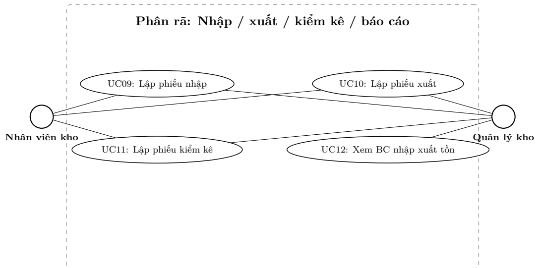
Figure 1: Use case phân rã – Nhập, xuất, kiểm kê, báo cáo tồn
